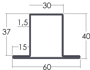
PILASTRA 40X30 (PDS41) Peso: 2,25 kg/m
