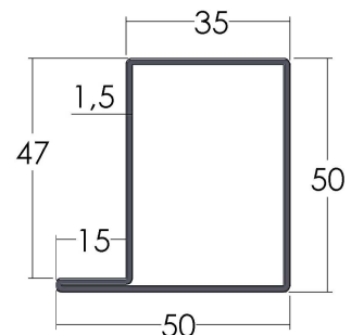
PILASTRA 40X30 (PDS28) Peso: 2,51 kg/m
